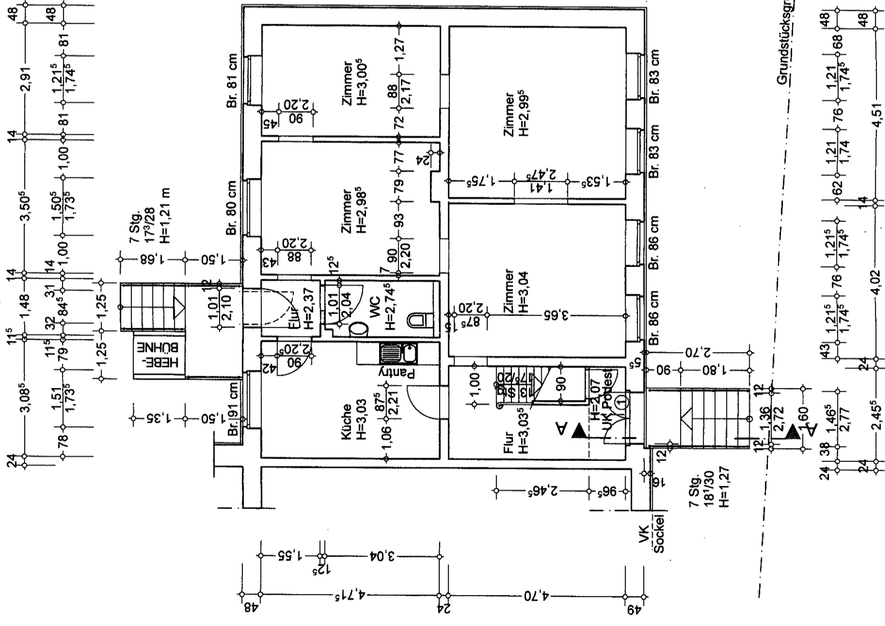
Grundriss Erdgeschoss Masstab 1:100
